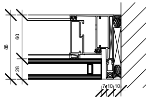
4 Detail 2 1 : 5
