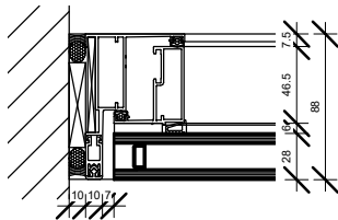
3 Detail 1 1 : 5
