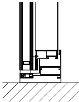
6 Detail 4 1 : 5
