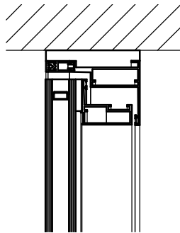
5 Detail 3 1 : 5
